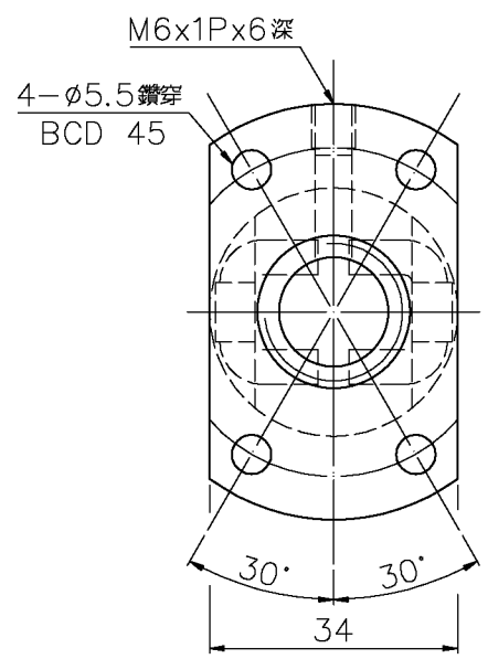
D-D 視圖
